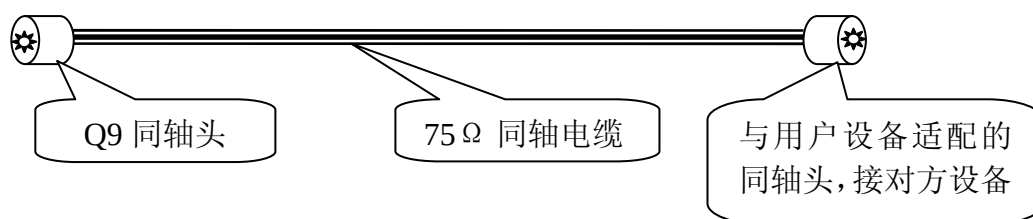
附图 2 HS-OPT101 光端机的 E1 接口连线制作方法
