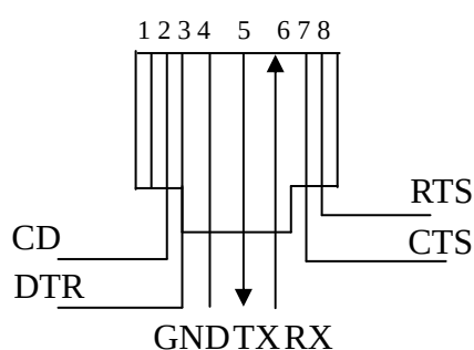
图 7.4 扩展串口接口定义
