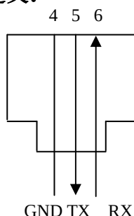
图 7.3 管理口 RS-232 接口定义
