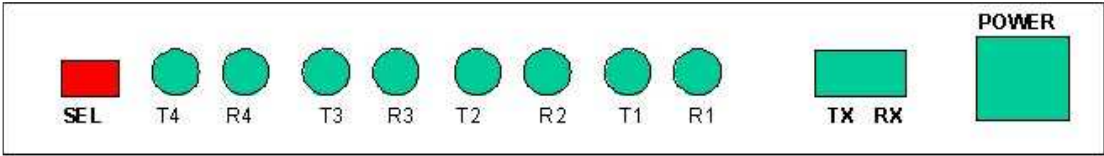
图 5.2 HS-OPT101 光端机后面板示意图(220V)
