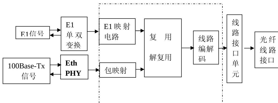
图 3.1 原理框图
