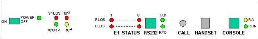
图 5.3 HS-OPT102 光端机前面板示意图
