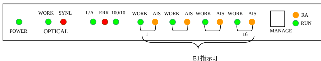
图 5.4: HS-OPT102E 前面板示意图
