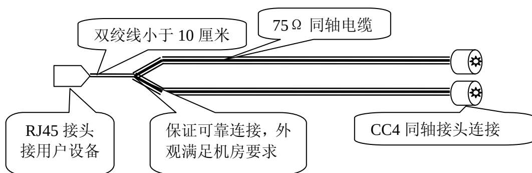
附 5 同轴接口与 RJ45 接口连接的 E1 接口连线制作方法
