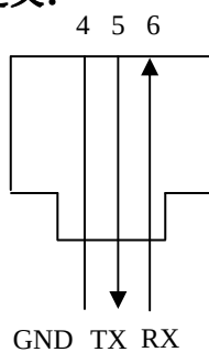
图 7.4 管理口 RS-232 接口定义
