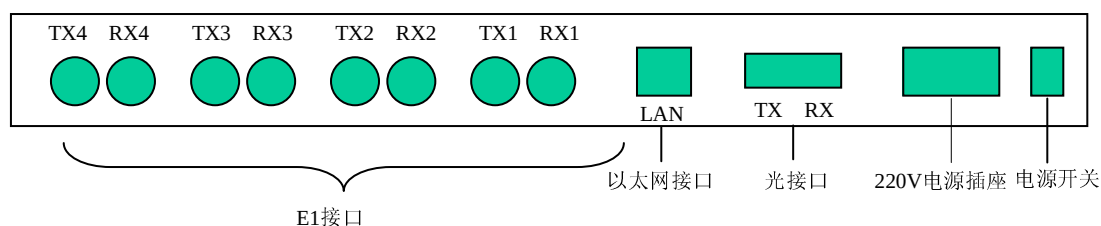
图 5.5: HS-OPT102E 后面板示意图
