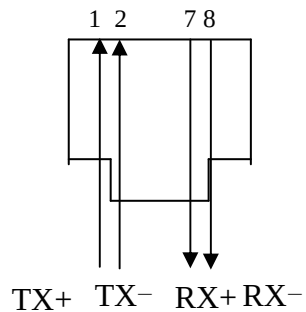
图 7.2 E1 接口 (RJ45) 定义
